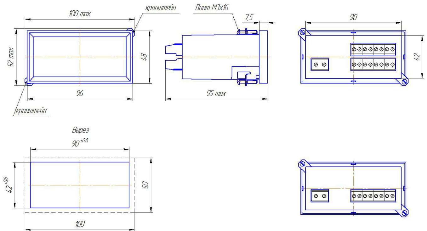
Рисунок А.2 – Общий вид, габаритные и установочные размеры приборов ЩЧ01П
