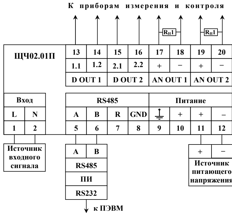
Рисунок Б.3 – Схема подключения приборов ЩЧ02.01П
